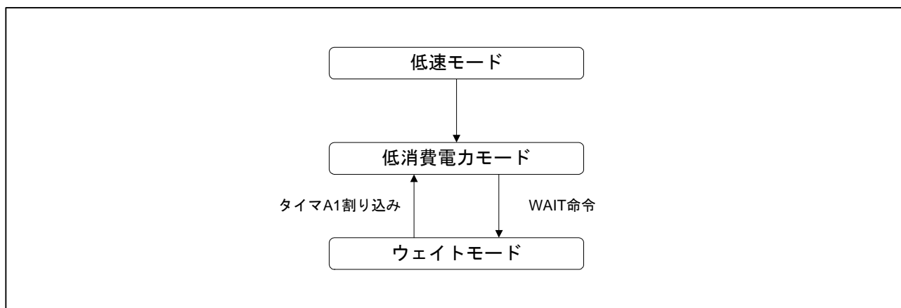
図 6 参考プログラムの状態遷移図
