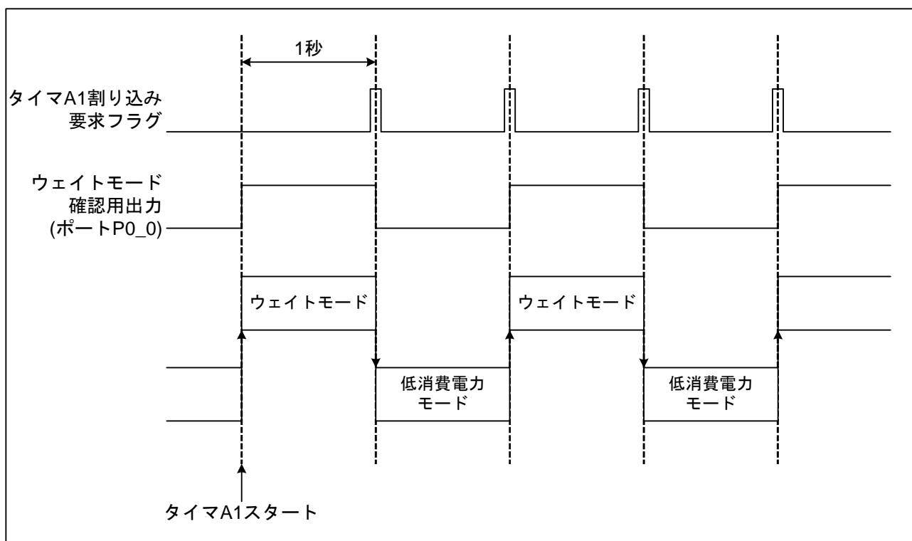
図 7 参考プログラムの動作イメージ
