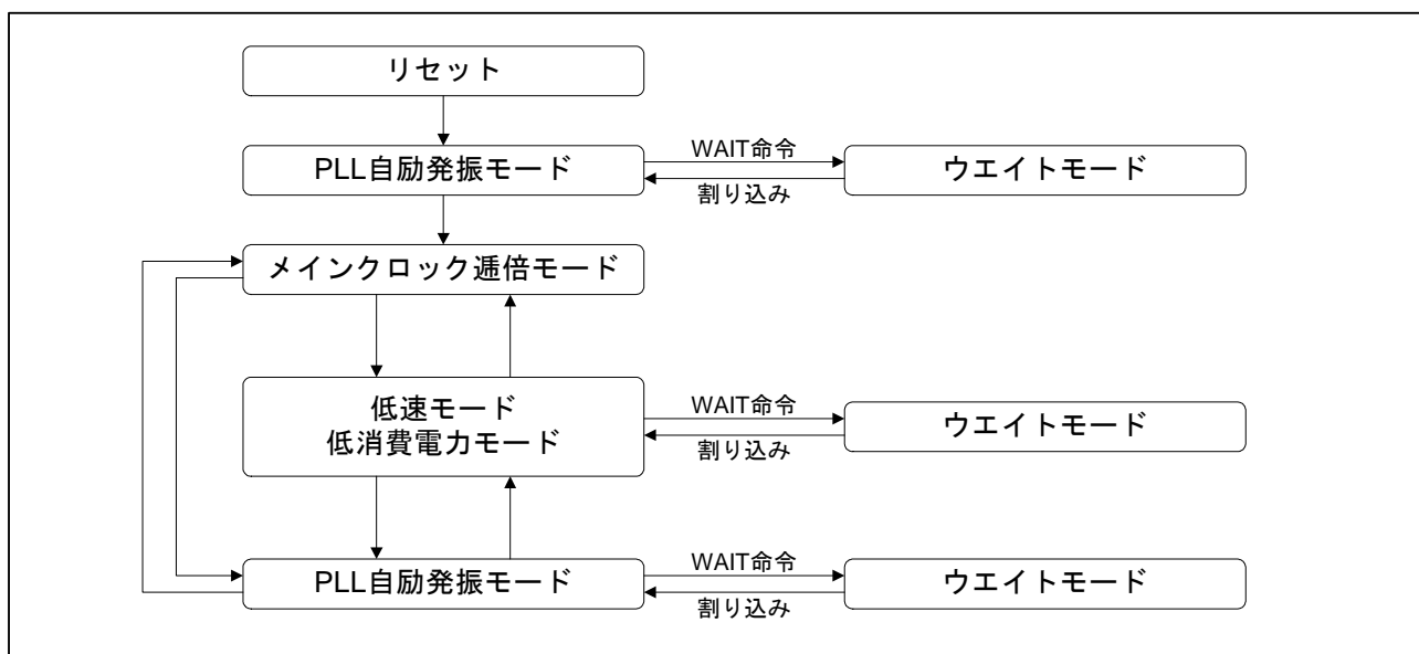
図 1 ウェイトモードへの状態遷移図
