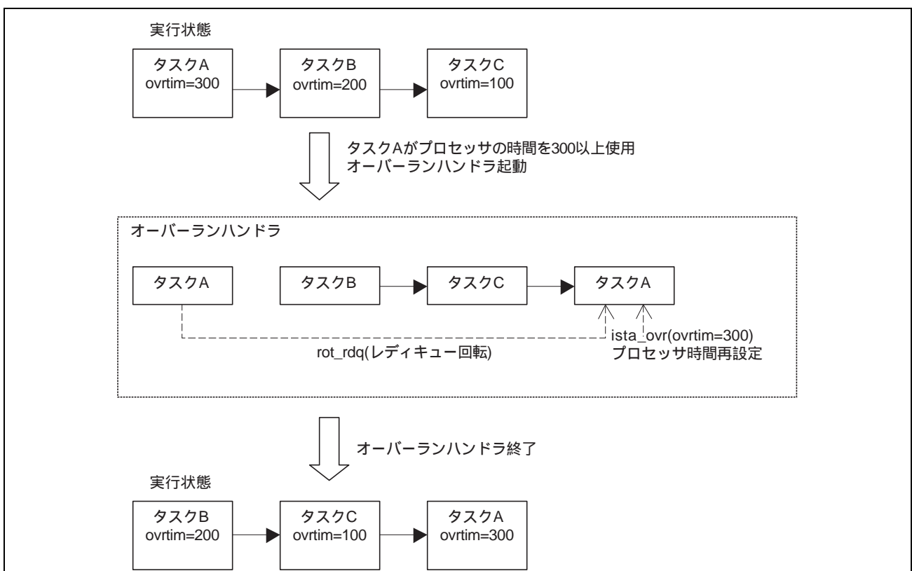
図 3-1 オーバーランハンドラ機能によるタイムスライス機能実装例
