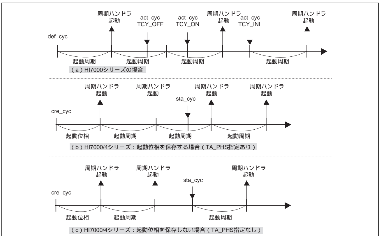
図 3-11 周期ハンドラの動作の違い
