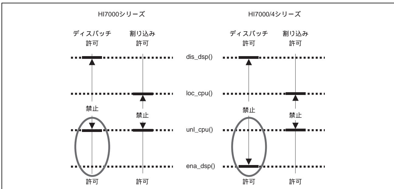
図 3-2 ディスパッチ禁止とCPUロックの変更
