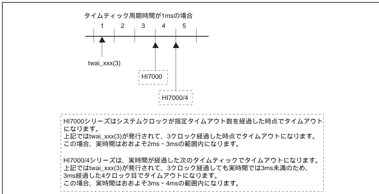
図 3-10 HI7000 シリーズと HI7000/4 シリーズの時間管理の違い
