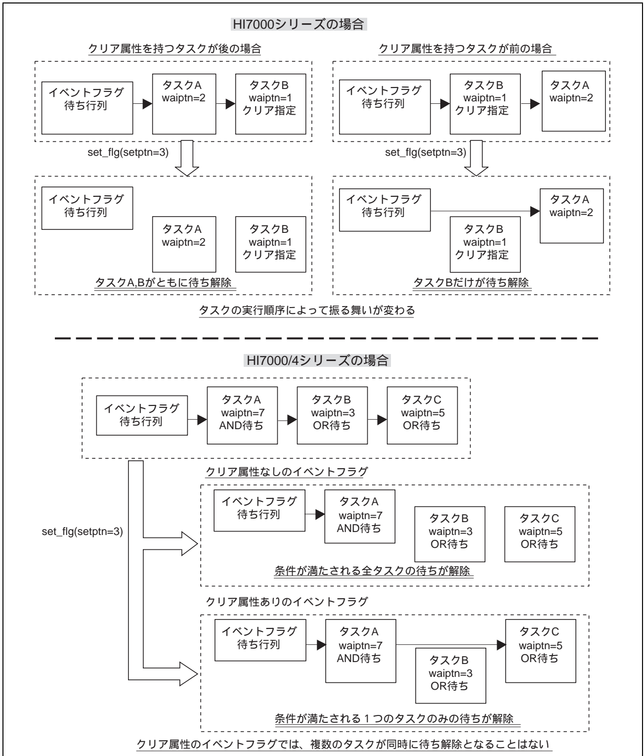
図 3-5 イベントフラグのクリア指定変更
