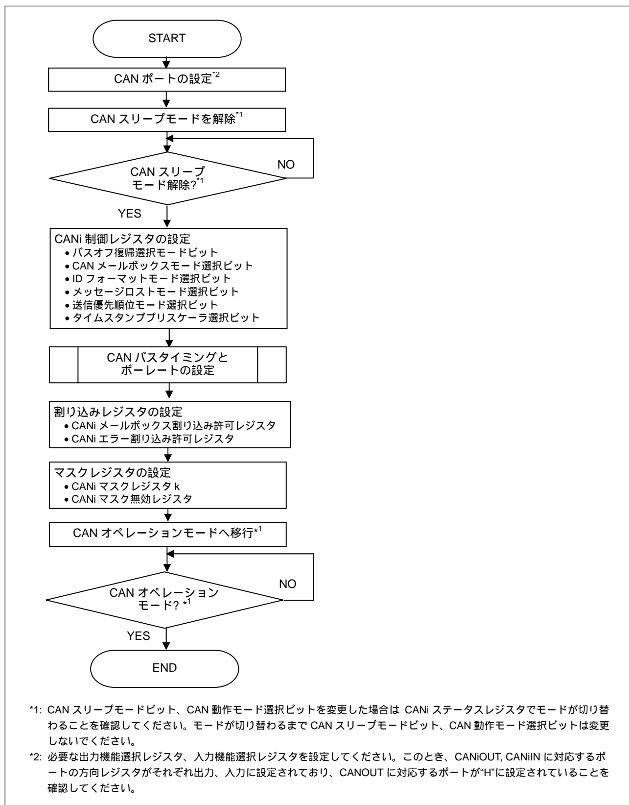
図 4 . ハードウェアリセット後に行う CAN コンフィグレーション手順
