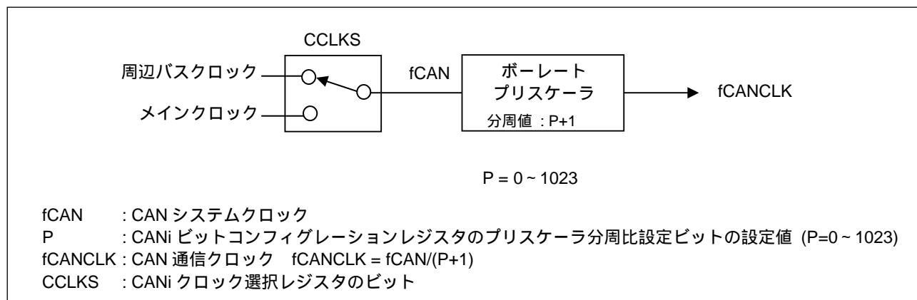
図 2 . CAN システムクロックの発生回路ブロック図
