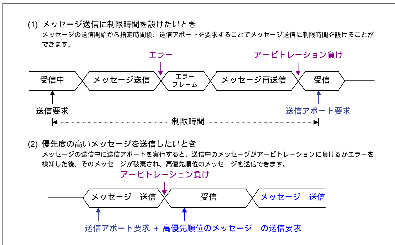
図 11. 送信アボート機能の応用例
