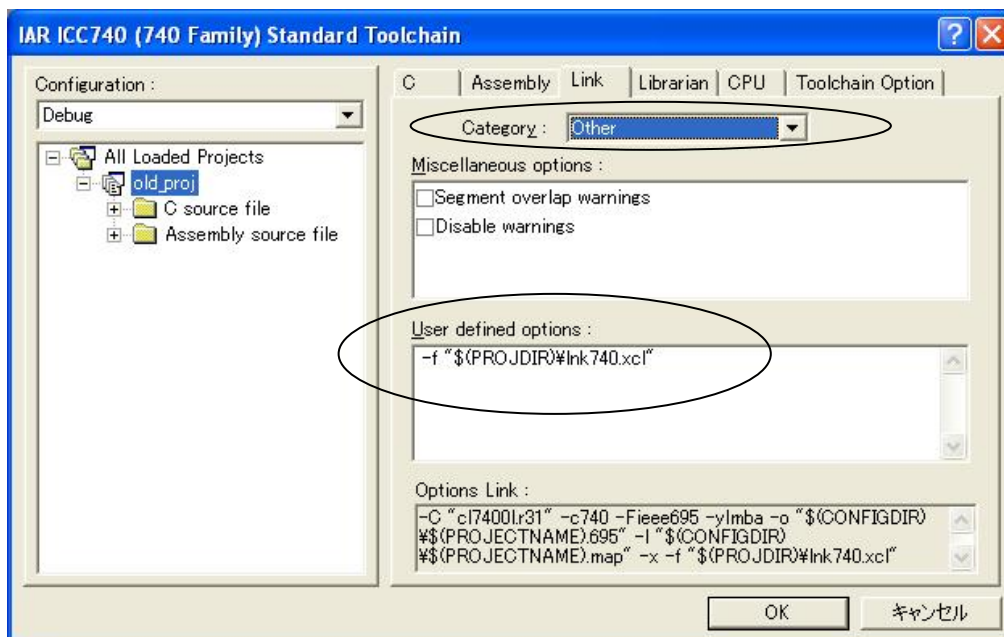
図 34 : ツールチェイン変更後の lnk740.xcl ファイルの設定箇所
