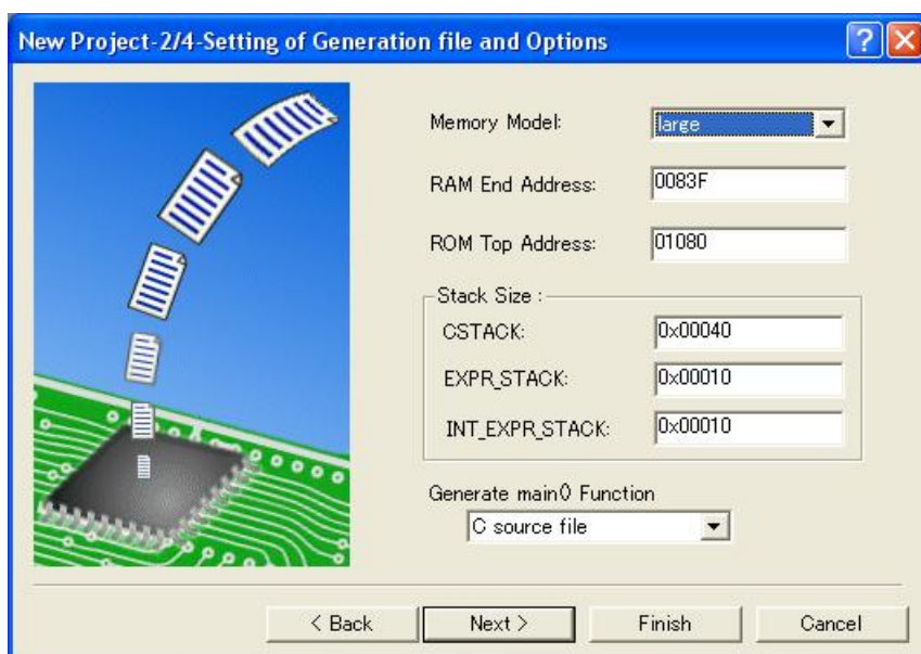
図 18 : [New Project]ウィザード : ステップ 2
