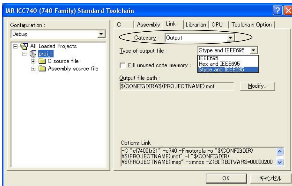
図 32 : [Toolchain]ダイアログボックスの Link タブの Category:Output
