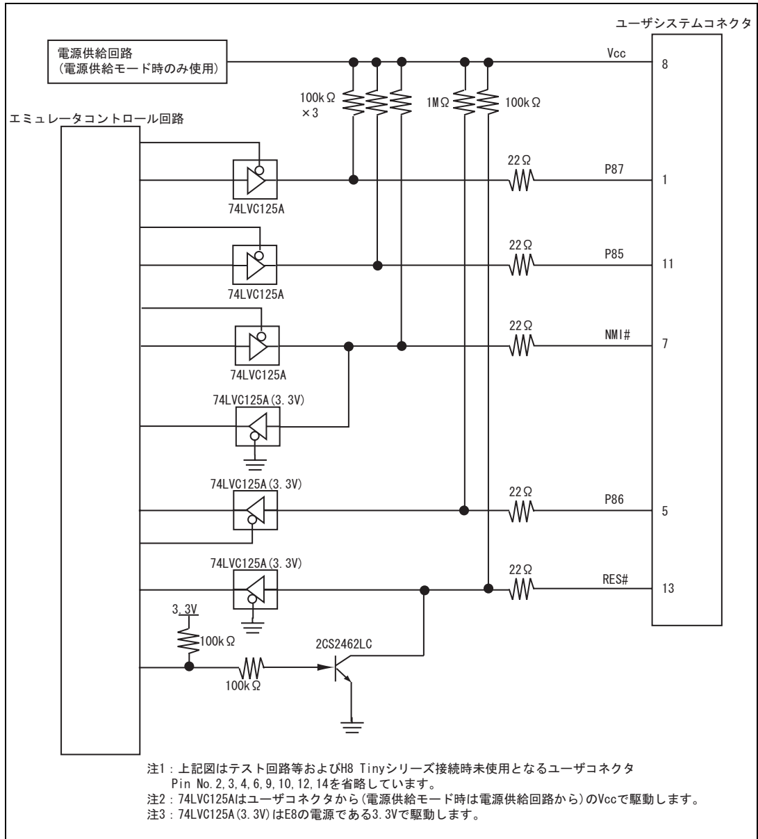
図 4.6 E8 エミュレータ内インタフェース回路 (参考)
